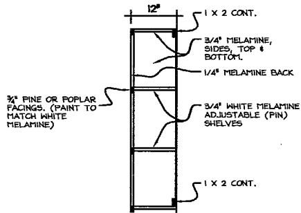
SECTION SCALE: 3/4" = 1'-0"
